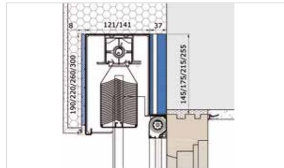
Mit Wärmedämmverbundsystem und Sturzdämmung RAFF S WDVS mit integriertem Rollo
